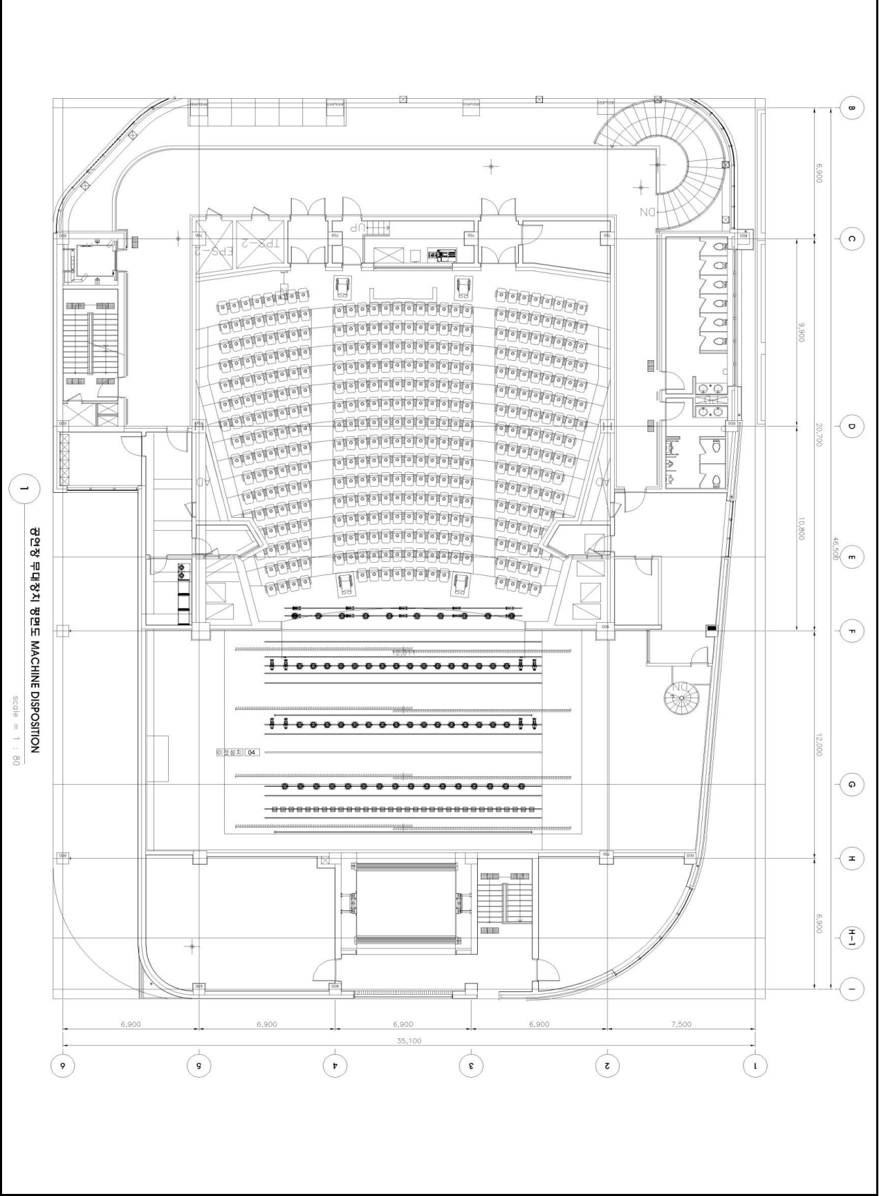
무대 평면도
