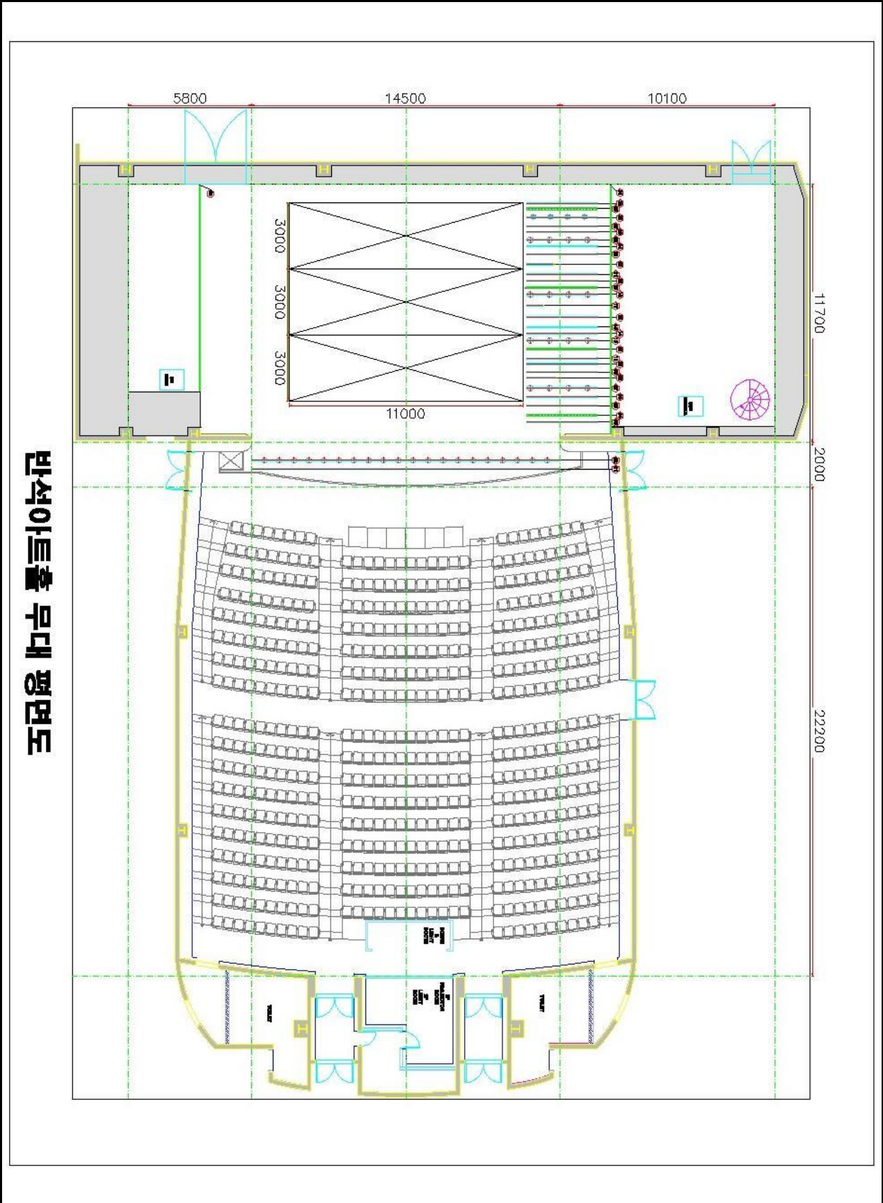
무대 평면도
